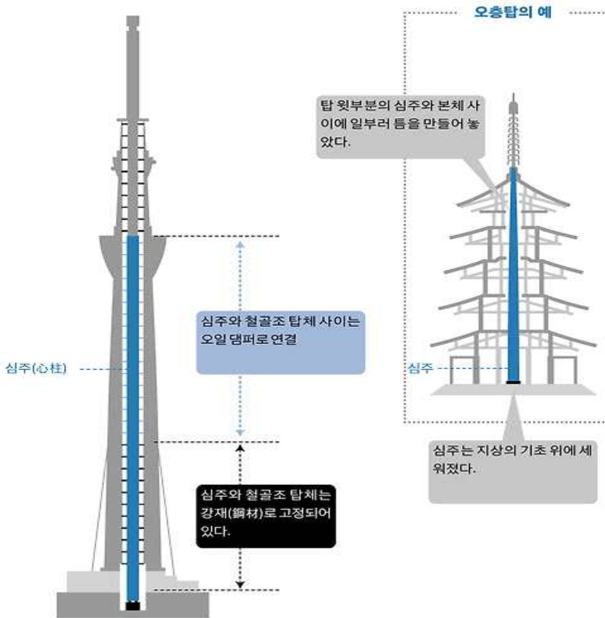
[도쿄 스카이트리 구조]
